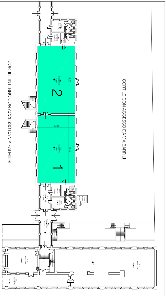
ESTRATTO Pianta Piano Terra
